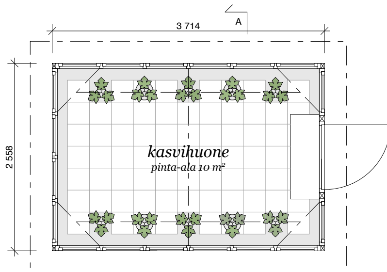
Pohjapiirros 1:50
