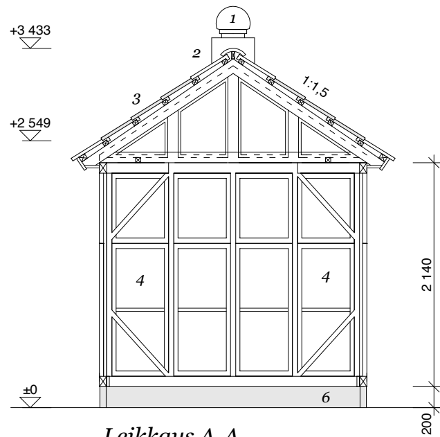
Leikkaus A-A
